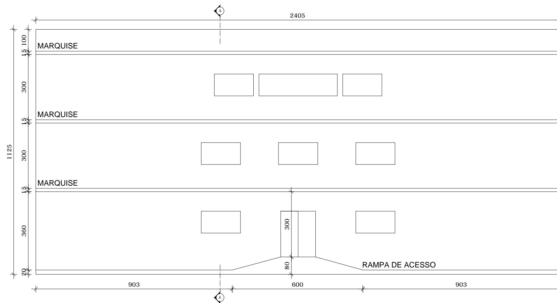
VISTA A ESC 1:100
