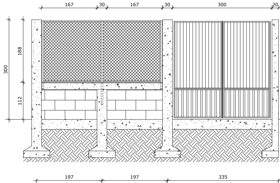
VISTA A ESC. 1/50
