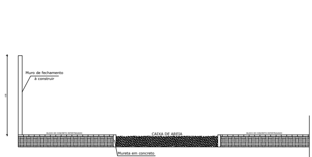
DETALHE 01 ESC. 1/50
