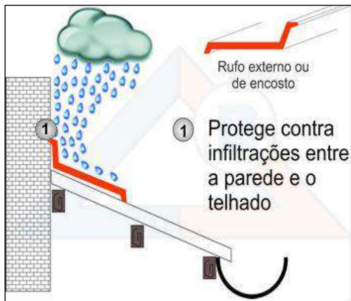
Detalhe de fixação de rufo, Pinterest 2024
