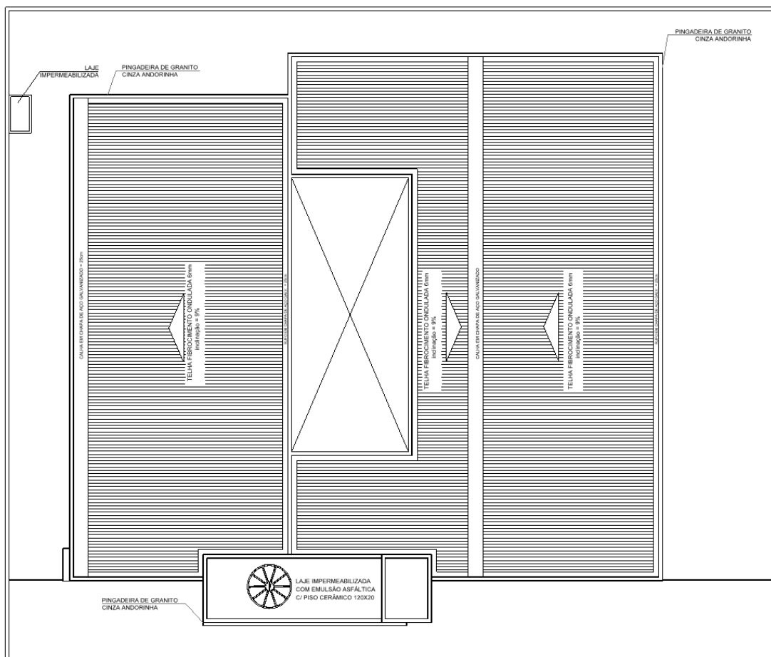
Figura 3 – Planta de cobertura da edificação.
