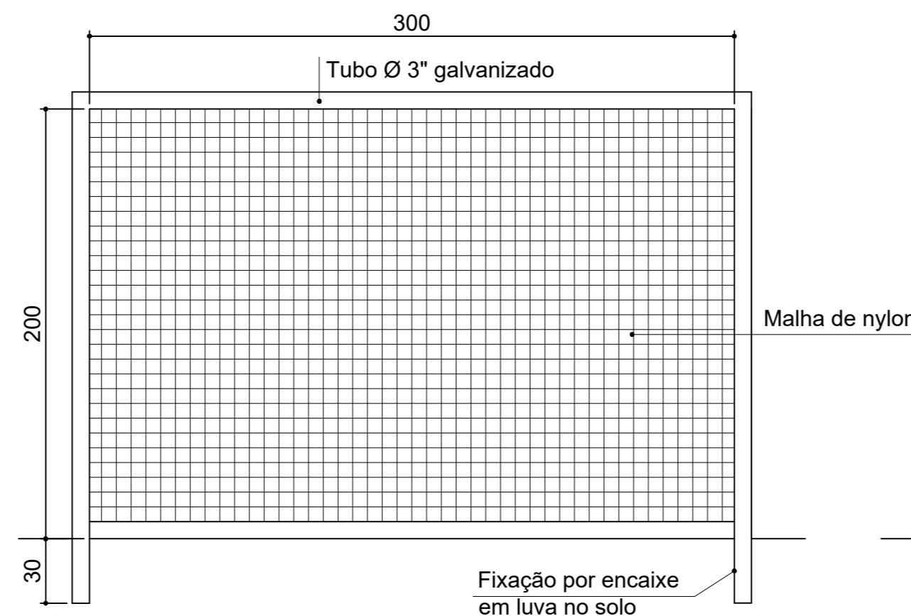
VISTA FRONTAL TRAVE Esc.: 1/25
