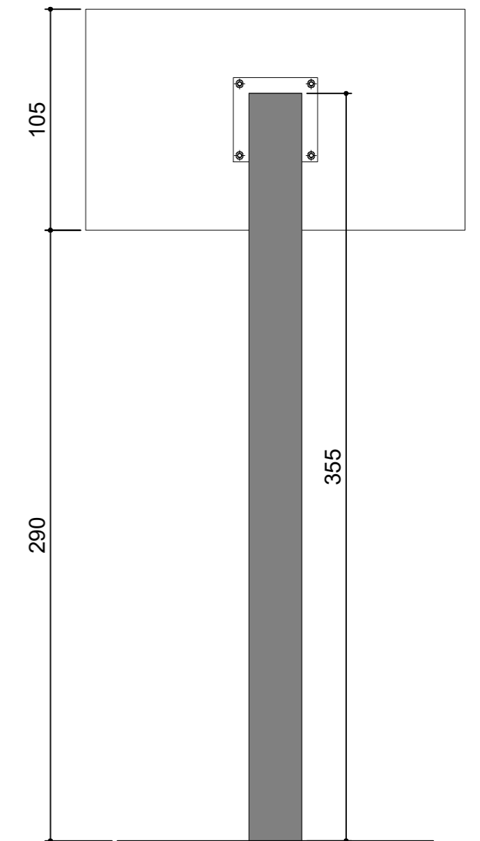
VISTA FUNDOS TABELA DE BASQUETEBOL Esc.: 1/25
