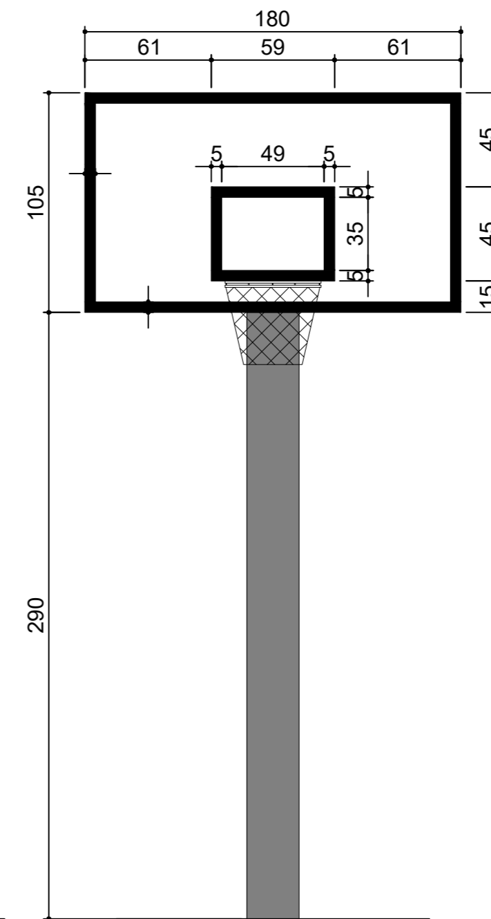
VISTA FRONTAL TABELA DE BASQUETEBOL Esc.: 1/25
