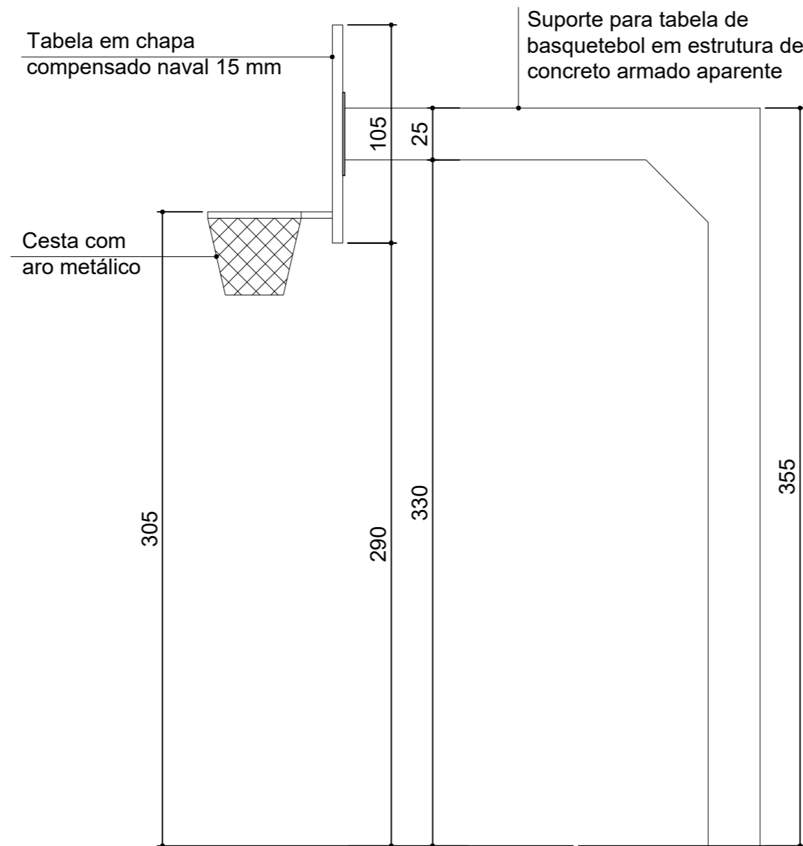
VISTA LATERAL TABELA DE BASQUETEBOL Esc.: 1/25
