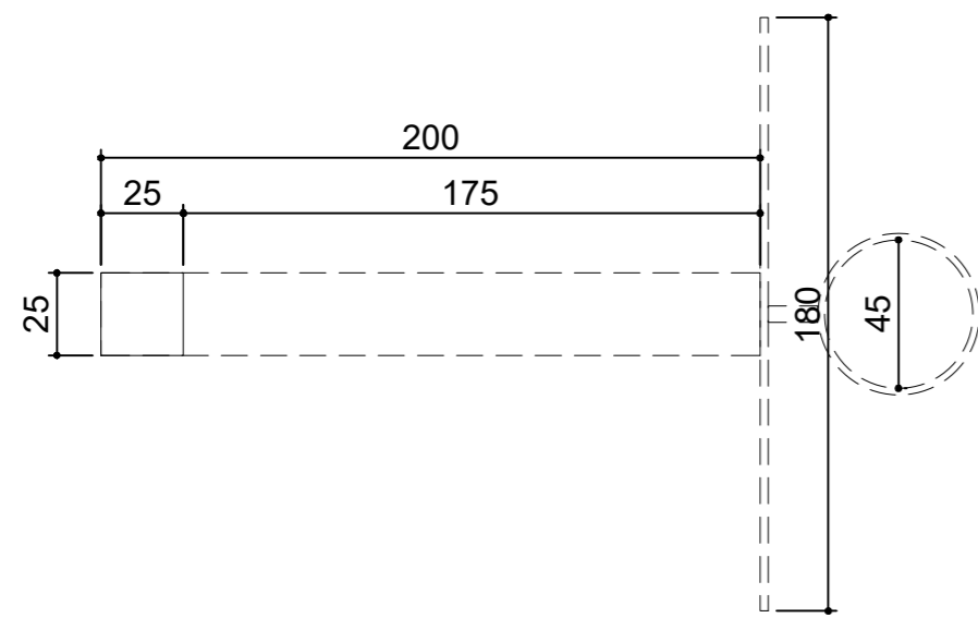
PLANTA BAIXA TABELA DE BASQUETEBOL Esc.: 1/25
