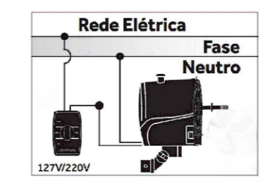
DETALHE ILUSTRATIVO ESQUEMA DE LIGAÇÃO DO VENTILADOR DE PAREDE SEM ESCALA
