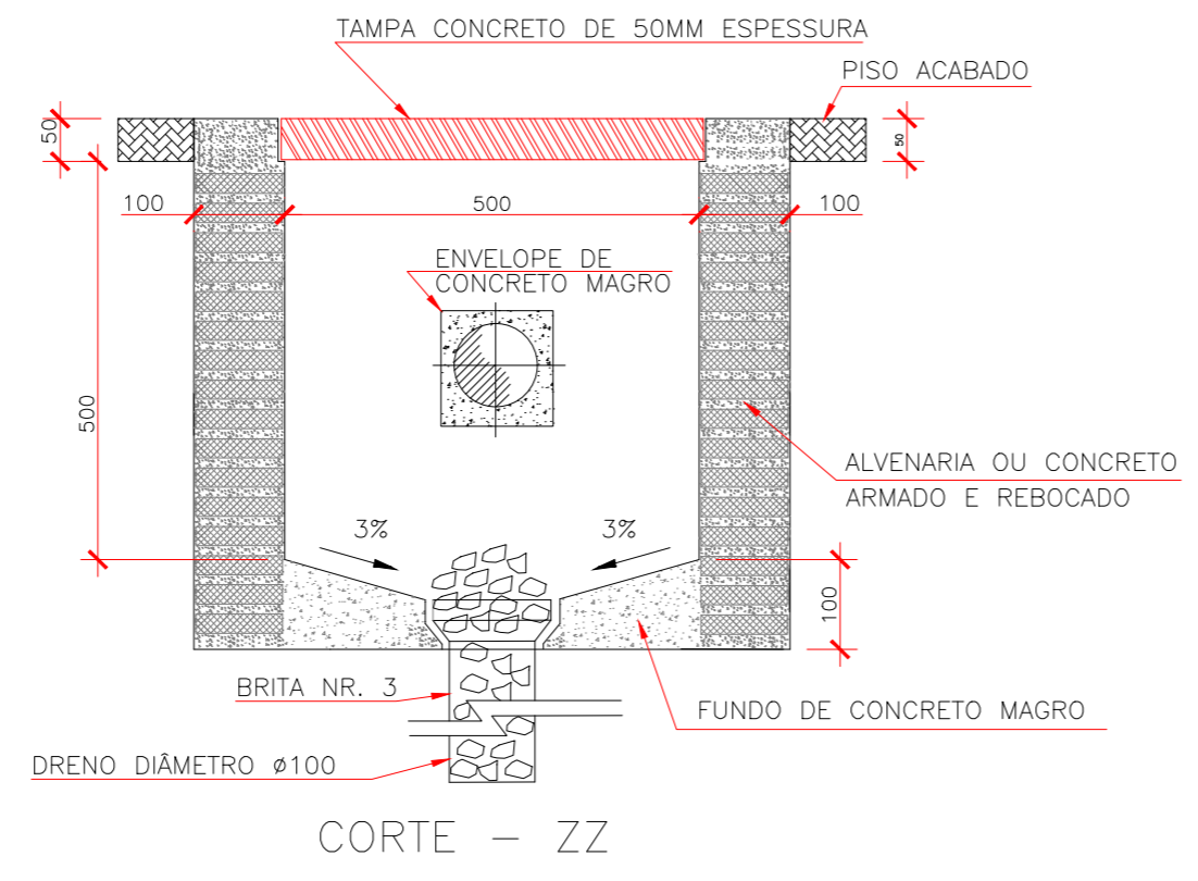
DETALHE 02 – CAIXA DE PASSAGEM 500X500X500 SEM ESC.
