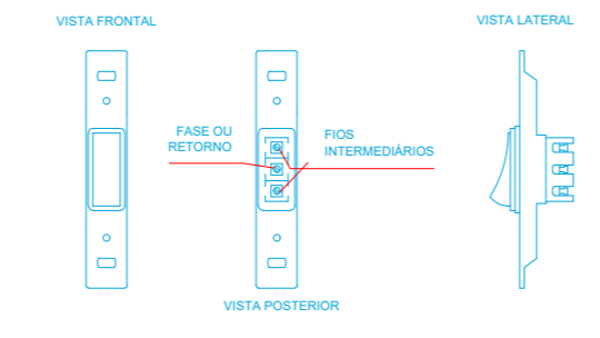
DETALHE ILUSTRATIVO INTERRUPTOR PARALELO SEM ESCALA
