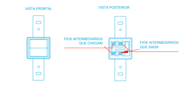
DETALHE ILUSTRATIVO INTERRUPTOR INTERMEDIÁRIO SEM ESCALA
