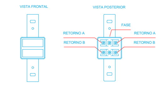
DETALHE ILUSTRATIVO INTERRUPTOR 2 TECLAS PARALELAS SEM ESCALA
