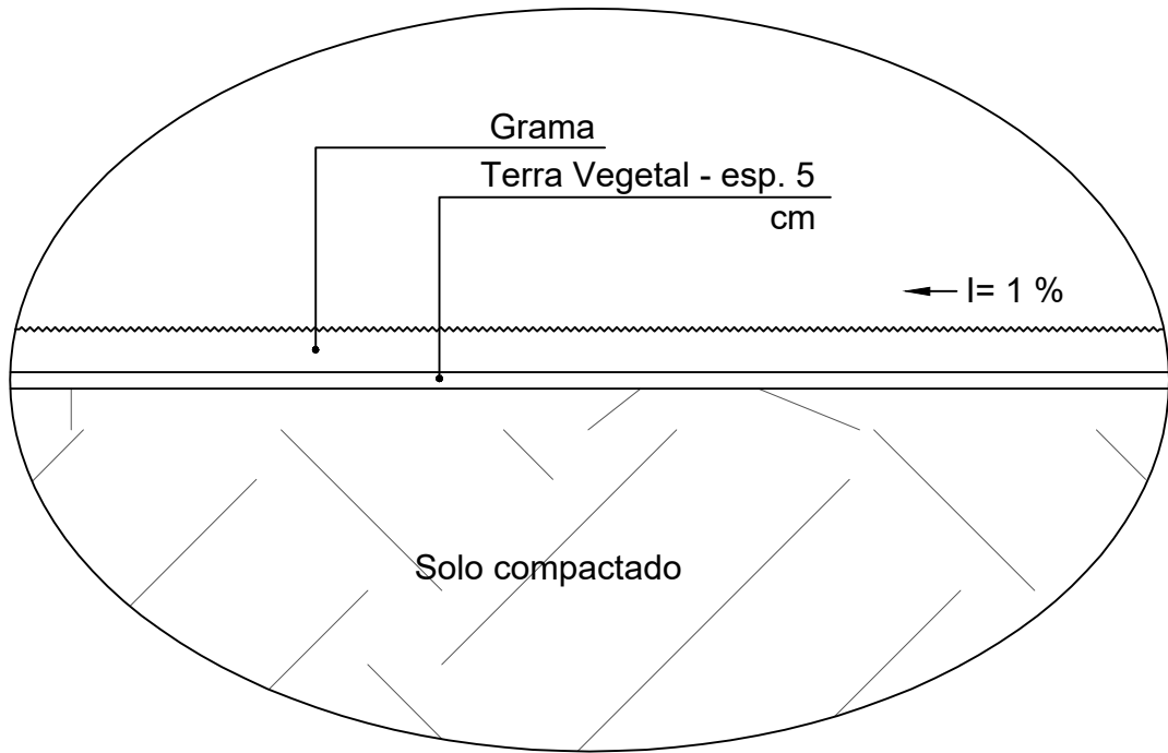
DETALHE GRAMADO
