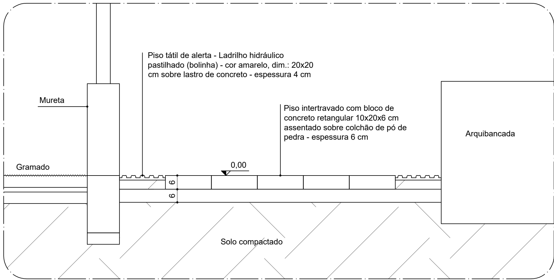
DET. 3 Esc.: 1/10
