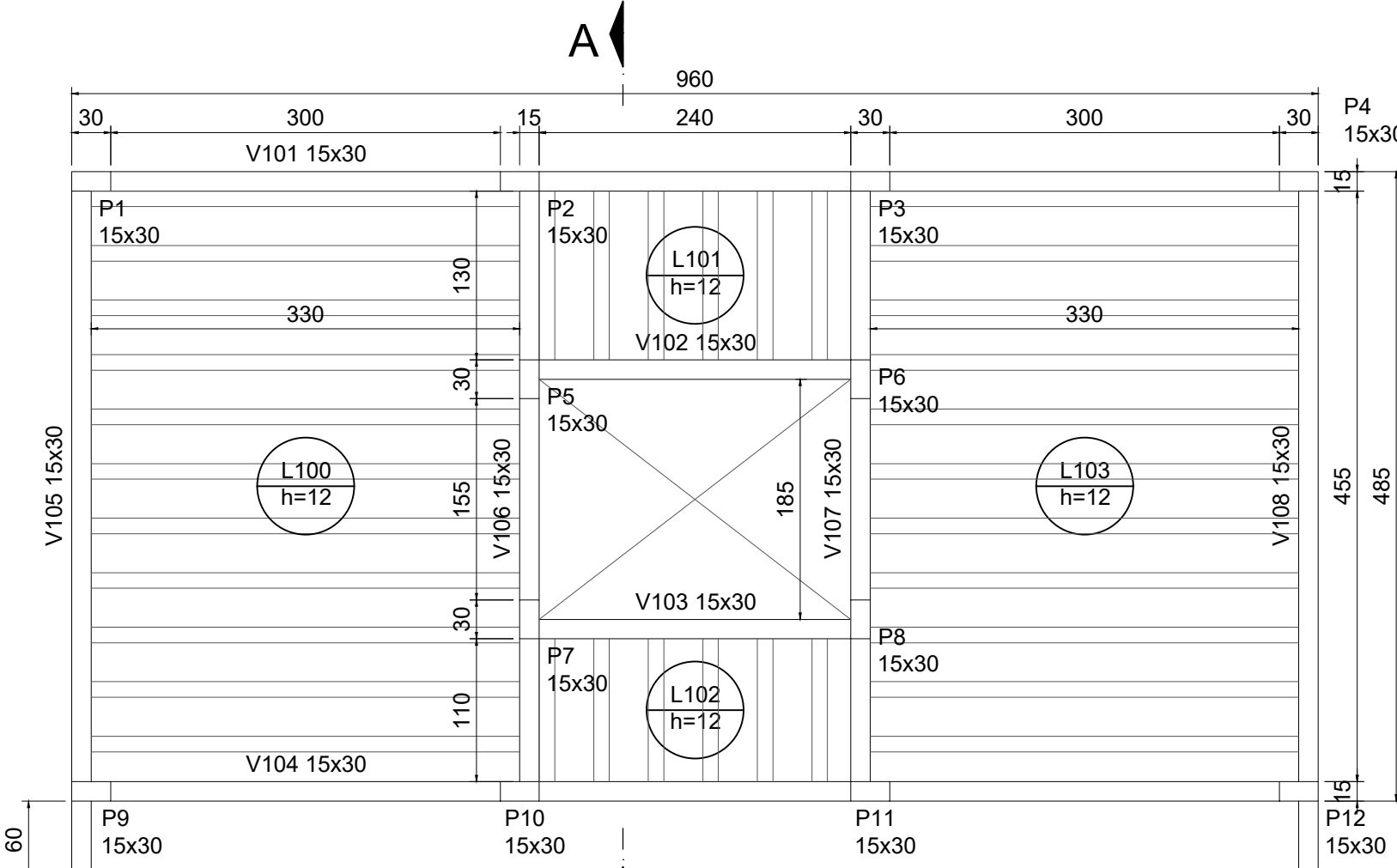
PLANTA DE FORMA - VIGAS (NÍVEL + 2,80) Esc.: 1/50
