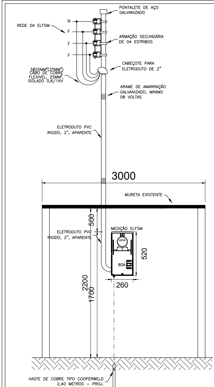
DETALHE 01 - REFORMA DE PADRÃO DE ENTRADA AÉREA EXISTENTE SEM ESCALA
