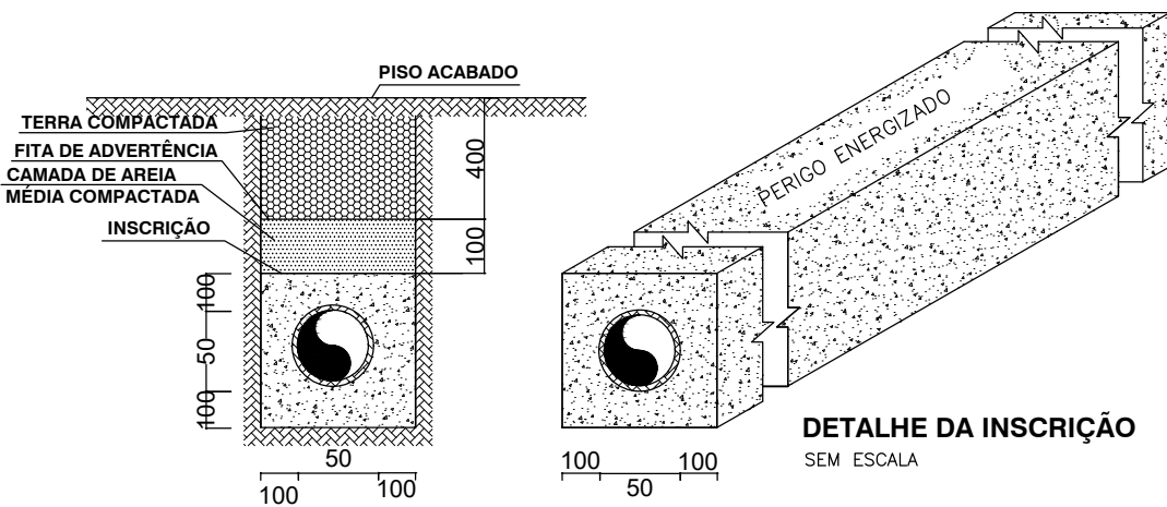
DETALHE 04 - ENVOLVIMENTO SEM ESCALA
