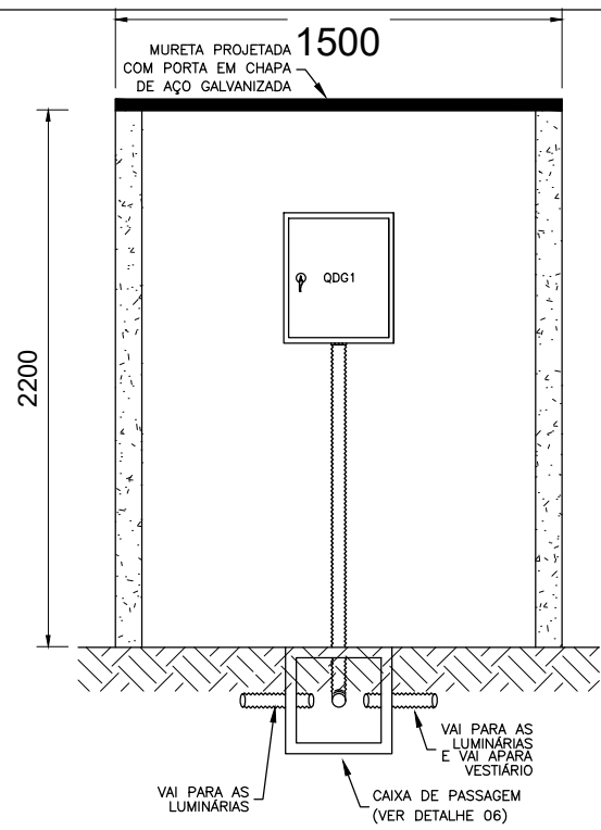
DETALHE 02 - MURETA PARA QUADRO GERAL DE DISTRIBUIÇÃO COM PORTAS DE AÇO GALVANIZADO. VISTA COM PORTAS ABERTAS SEM ESCALA
