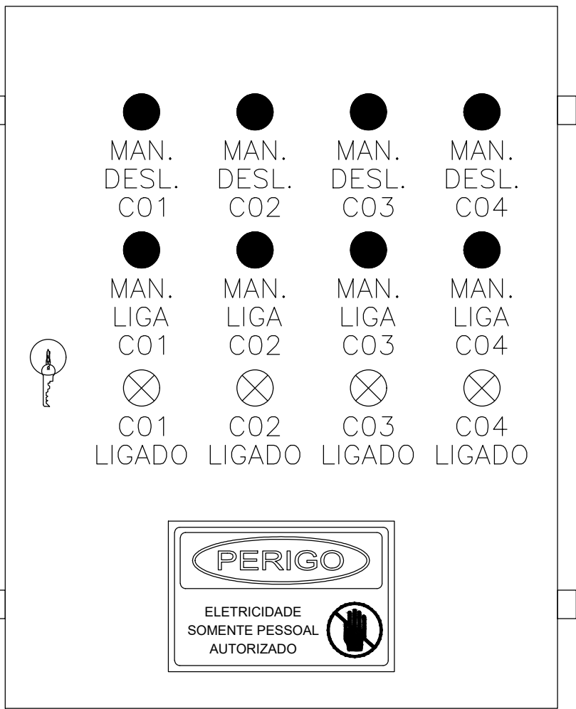
LAYOUT EXTERNO - PAINEL DE FORÇA E COMANDO DOS REFLETORES
