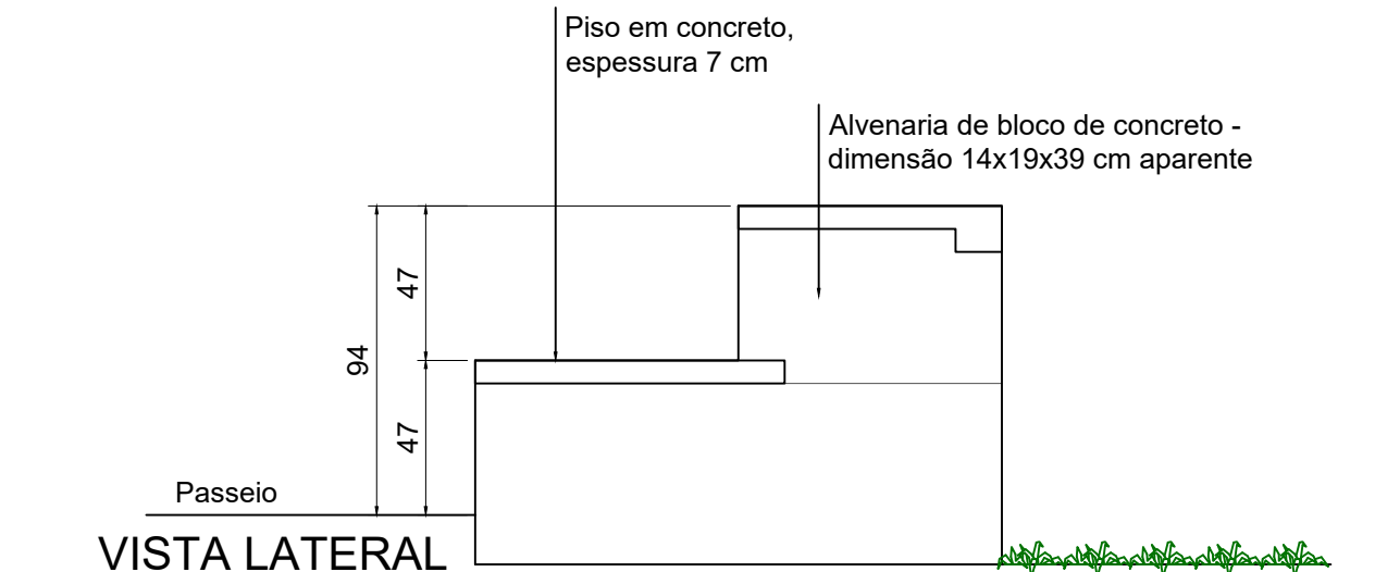
VISTA LATERAL
