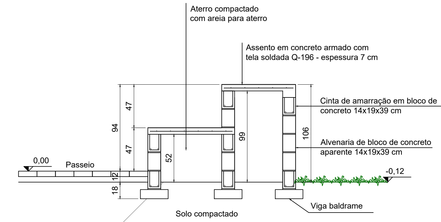
ESQUEMA ESTRUTURA ARQUIBANCADAS Esc.: 1/25
