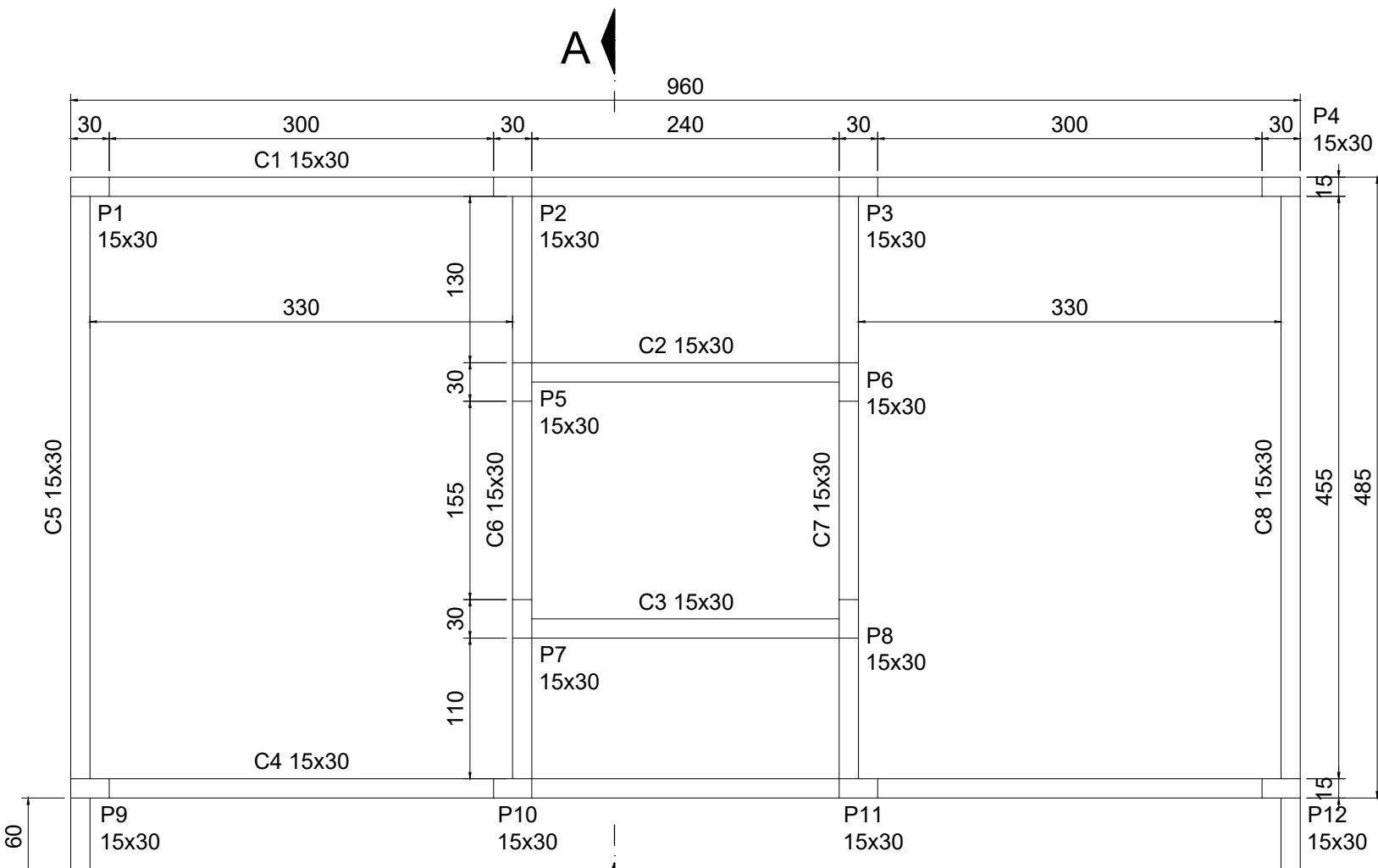
PLANTA DE FORMA - CINTAMENTO (NÍVEL 0,00) Esc.: 1/50
