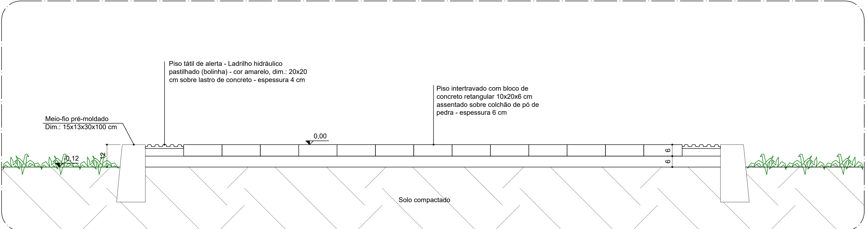
DET. 1 Esc.: 1/10
