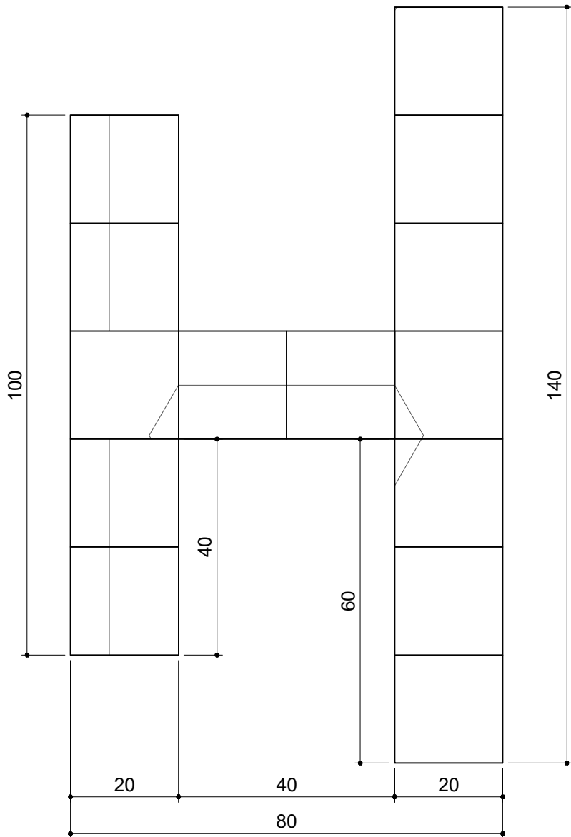
DET. 4 Esc.: 1/10
