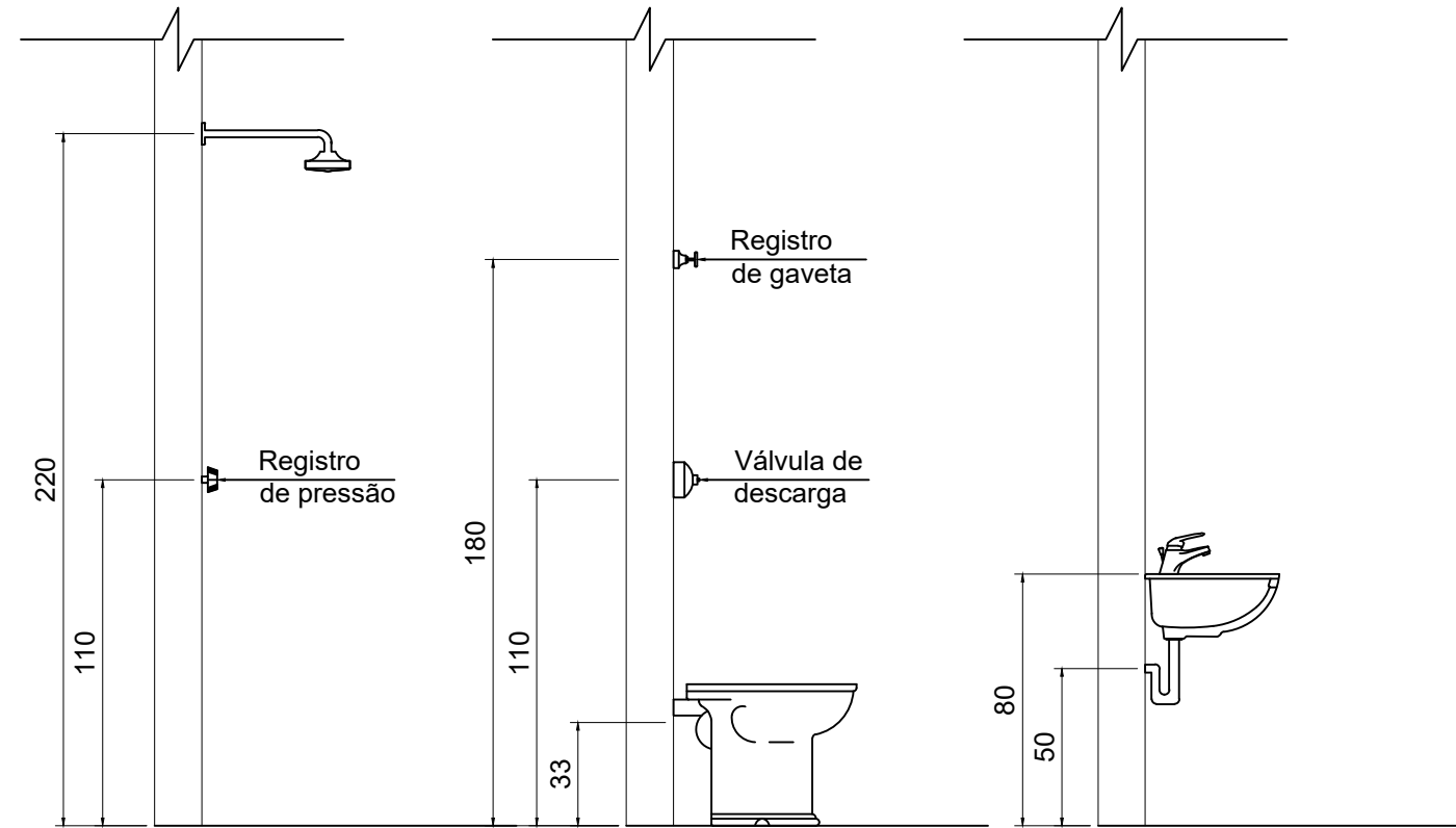
ALTURA PONTOS ACESSÓRIOS Esc.: 1/25
