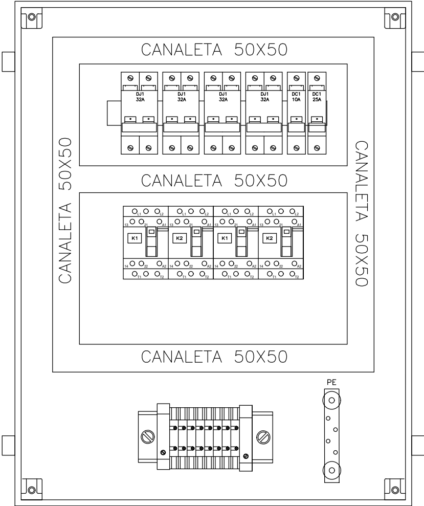
LAYOUT INTERNO - PAINEL DE FORÇA E COMANDO DOS REFLETORES
