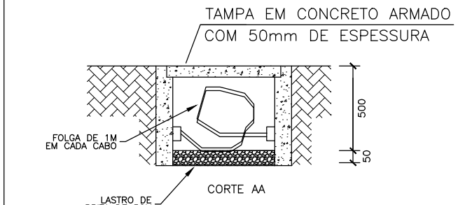
DETALHE 06 - CAIXA DE PASSAGEM SEM ESCALA
