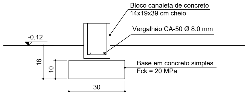
BASE ARQUIBANCADAS Esc.: 1/10
