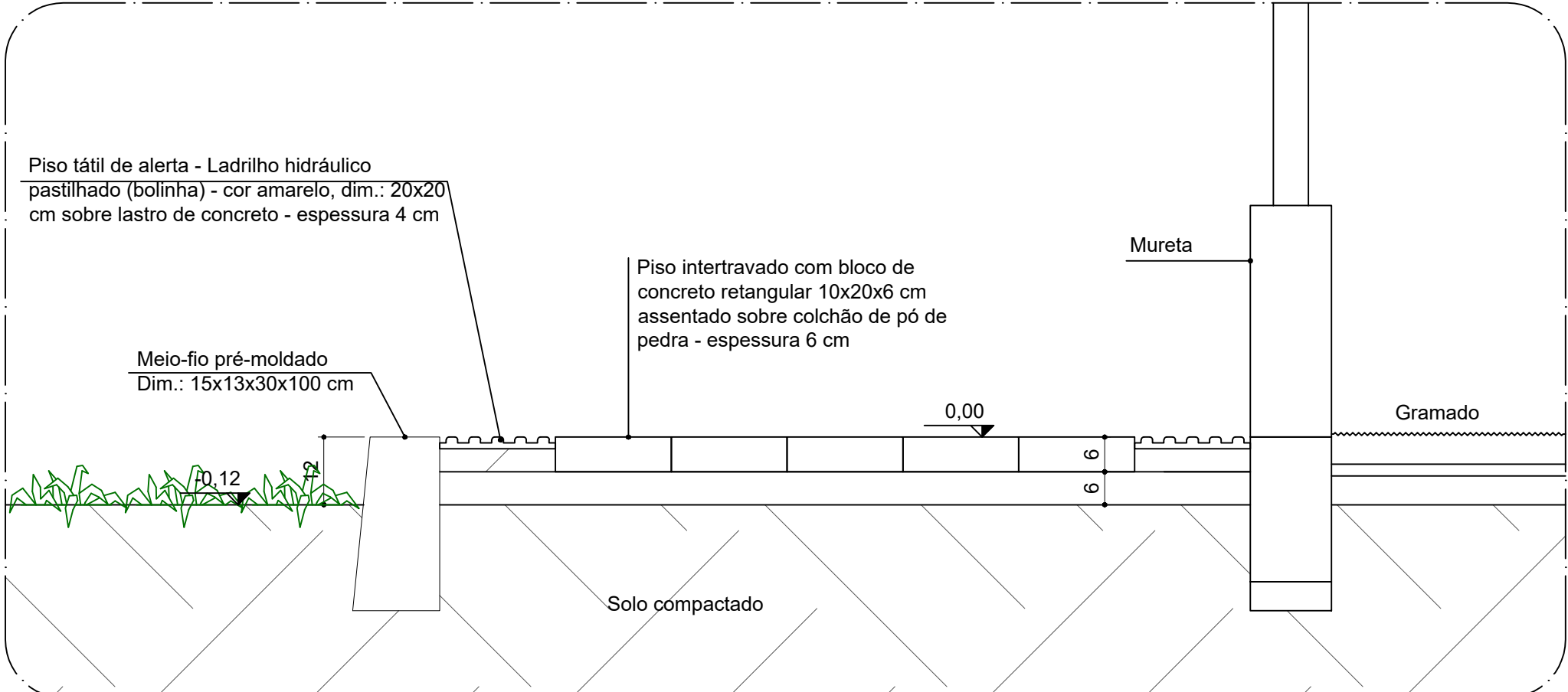
DET. 2 Esc.: 1/10
