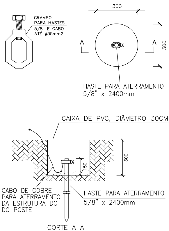
DETALHE 05 - CAIXA DE ATERRAMENTO SEM ESCALA
